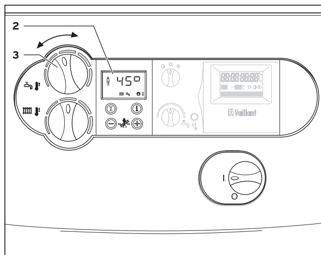
Fig. 4.6 Impostazione della temperatura serbatoio (solo con boiler collegato)
